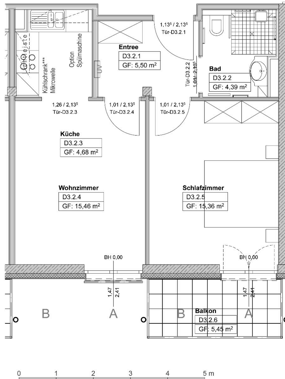
Wohnung D3.2 NGF 48,12 m 2 Balkonfläche nur zur Hälfte angerechnet
