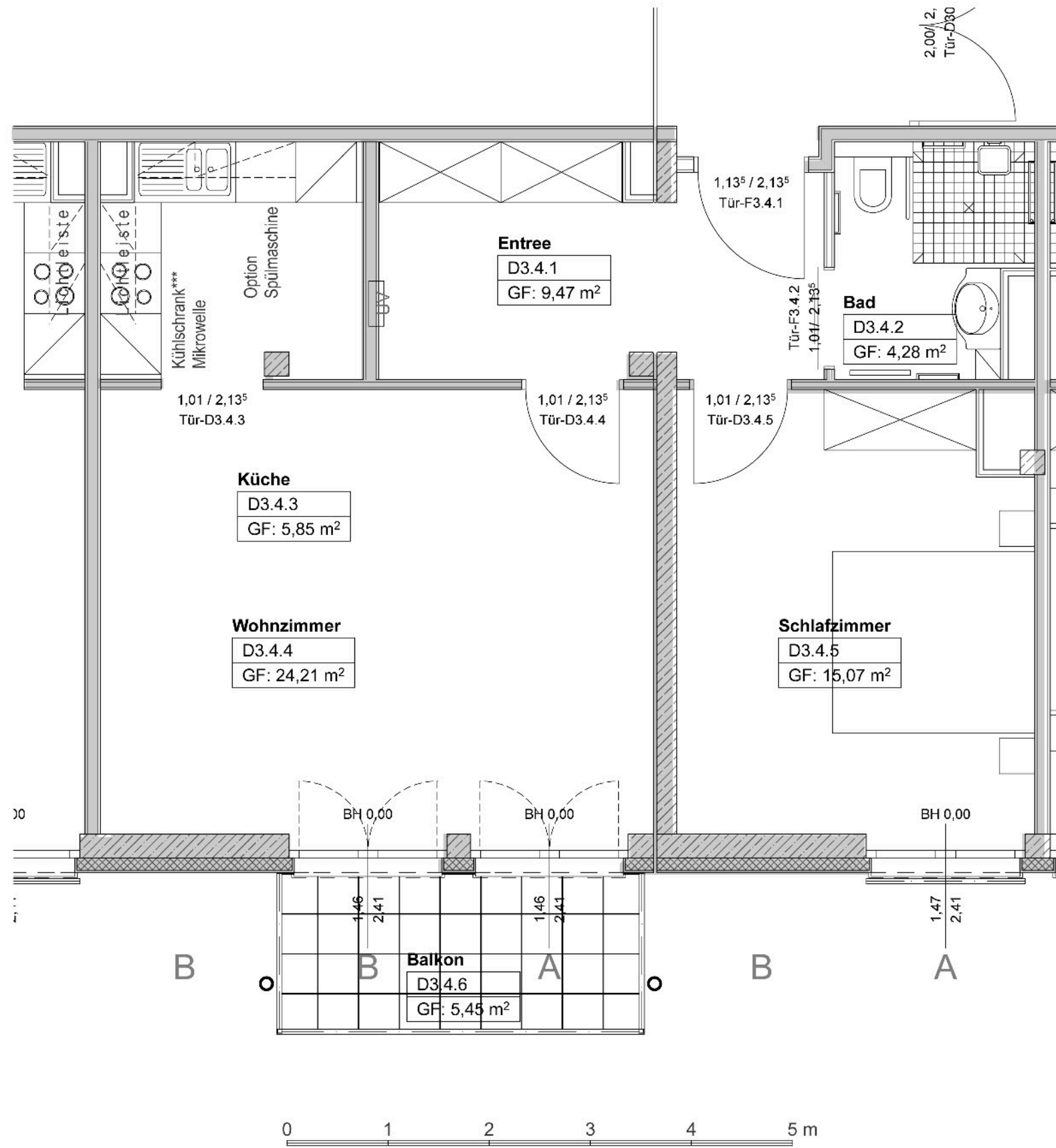
Wohnung D3.4 NGF 61,61 m 2 Balkonfläche nur zur Hälfte angerechnet
