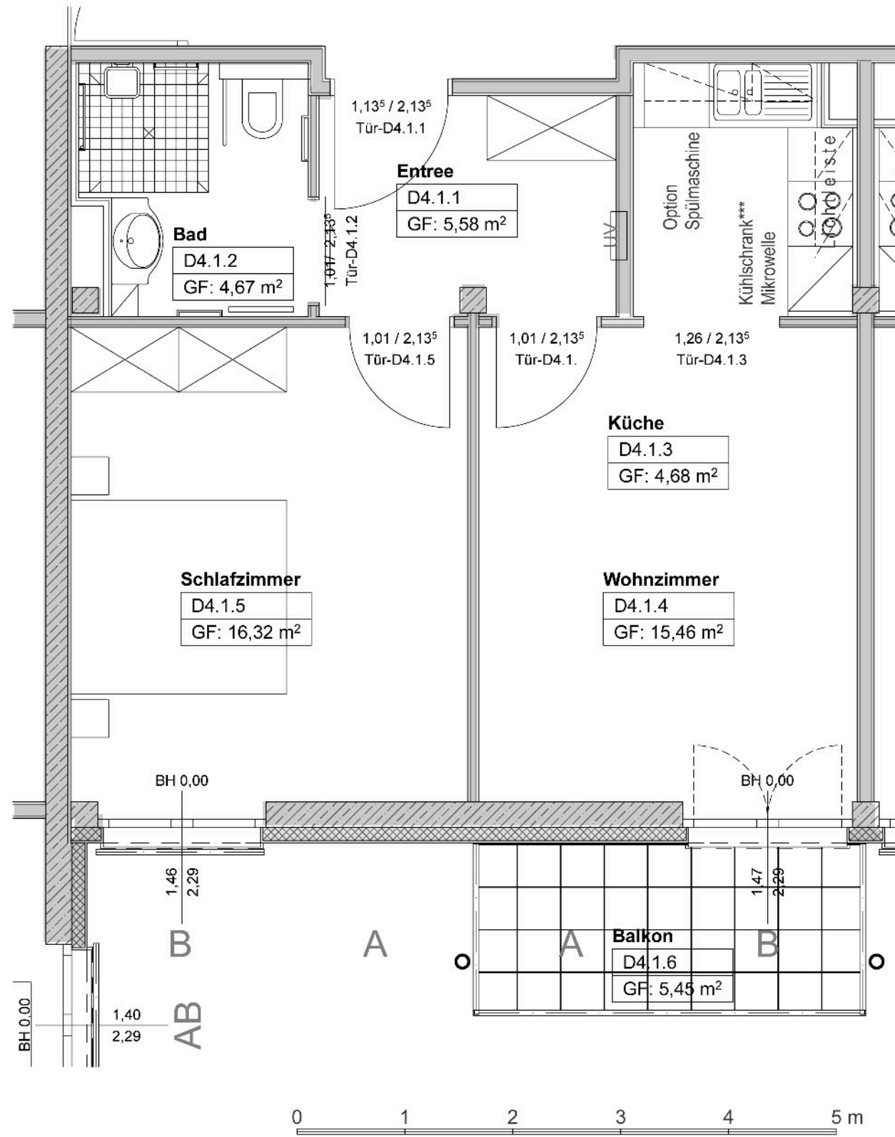
Wohnung D4.1 NGF 49,44 m 2 Balkonfläche nur zur Hälfte angerechnet
